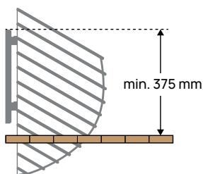
Rys. 6. Montaż pieca elektrycznego HUUM DROP wewnątrz ławki.
