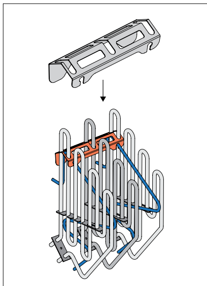
3. attēls HUUM DROP 4, 6 un 7 atdalītā-jrežģa uzstādīšana ar 3 sildelementiem.
