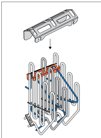
Slika 3 Instaliranje nosača za HUUM DROP 4, 6 i 7, s tri grijača elementa.
