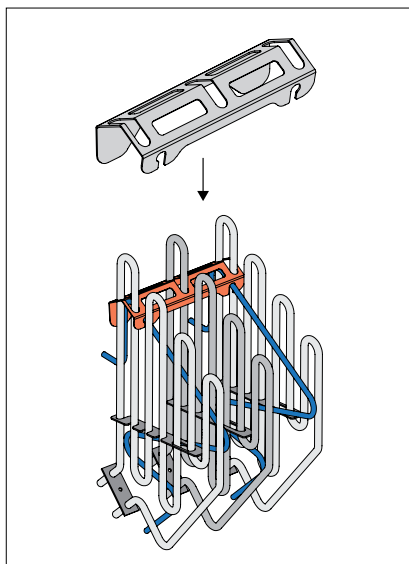
3 pav. HUUM DROP 4, 6 ir 7 su 3 kaitinimo elementais laikiklio montavimas.
