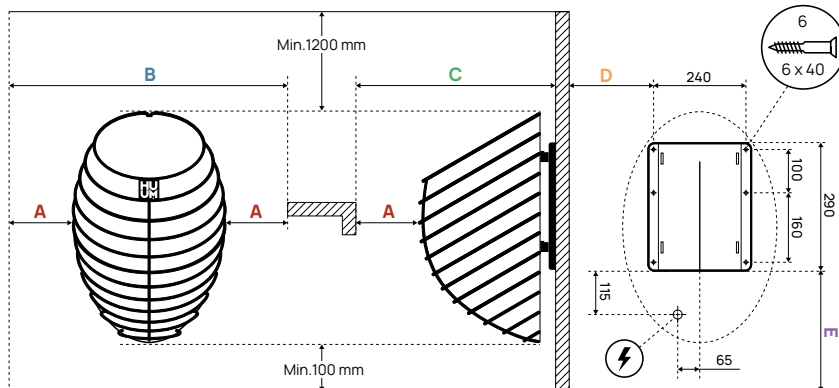
Rys. 1. Ustawianie pieca.
