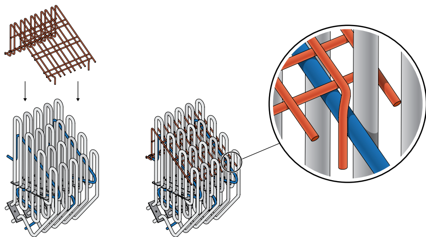
Rys. 5. Montaż uchwyty ustalającego HUUM DROP 9 z pięcioma elementami grzewczymi.
