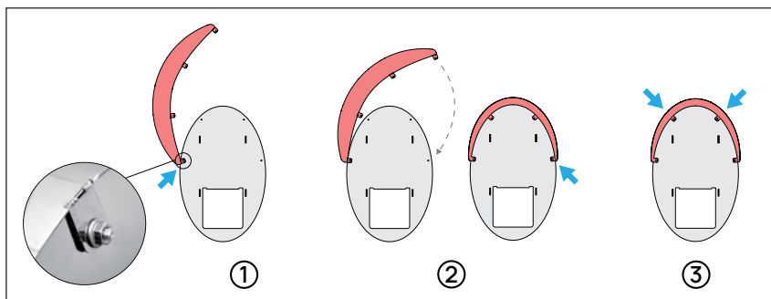
Rys. 2. Montaż rozpraszacza ciepła.
