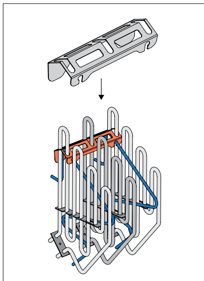
3. ábra: A HUUM DROP 4, 6 és 7 rögzítőjének felszerelése 3 fűtőelemmel.
