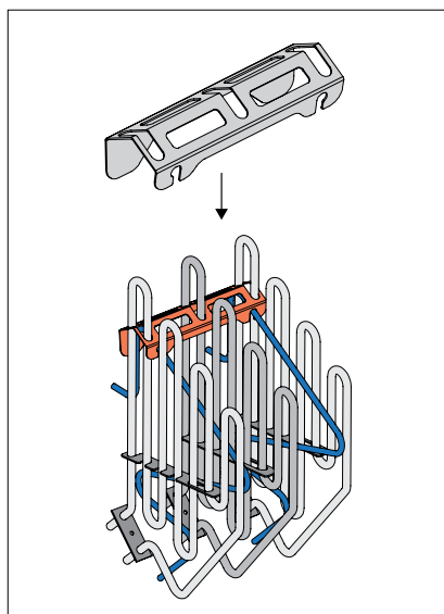
Rys. 3. Montaż uchwyty ustalającego HUUM DROP 4, 6 i 7 z trzema elementami grzewczymi.
