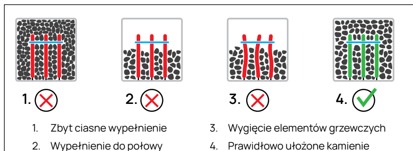
Rys. 7. Umieszczenie kamieni w piecu DROP 4, 6 i 7 z trzema elementami grzewczymi.
