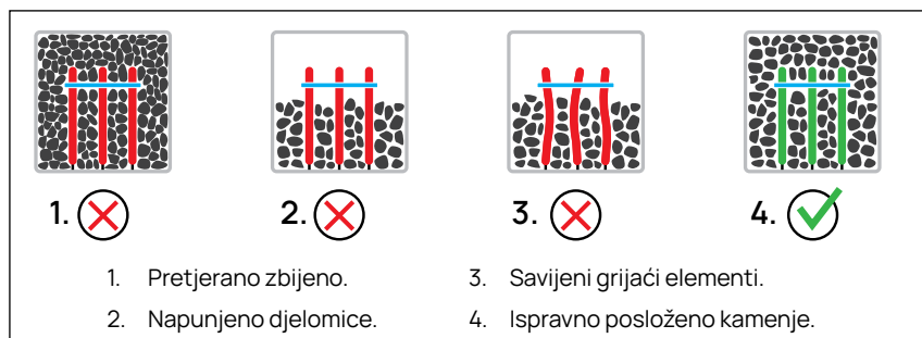
Slika 7 Postavljanje kamenja u DROP 4, 6 i 7, s tri grijaća elementa.
