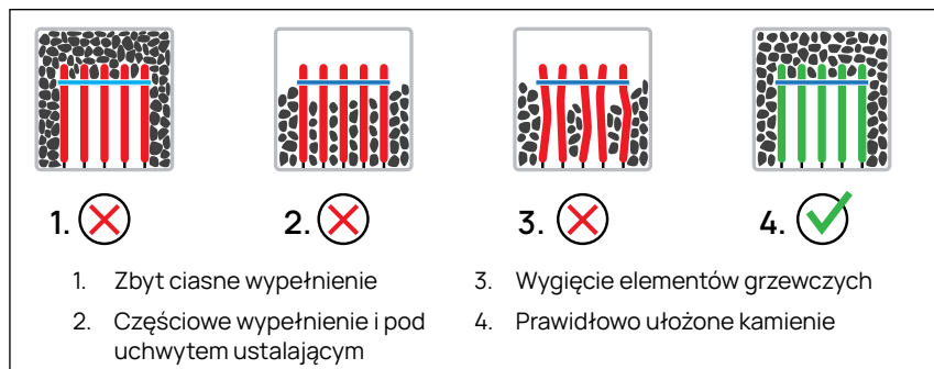
Rys. 8. Umieszczenie kamieni w piecu DROP 9 z pięcioma elementami grzewczymi.
