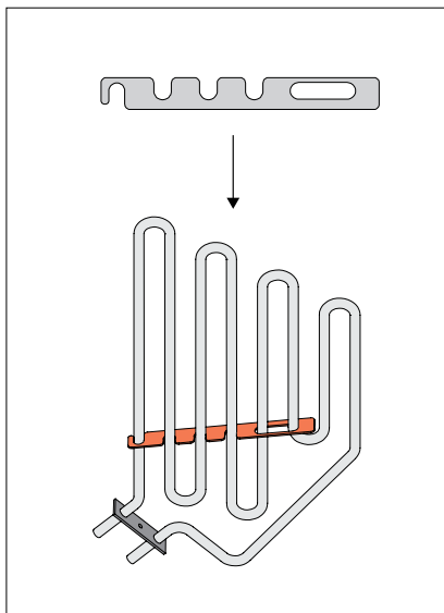
4. attēls HUUM DROP sildelementu fiksatora uzstādīšana.
