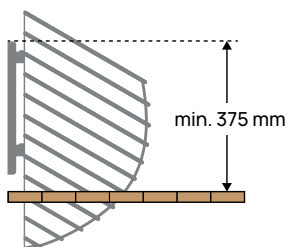
6. attēls HUUM DROP elektriskās krāsns iegremdēšana pirts lāvā.
