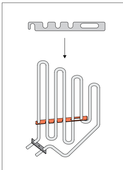
Rys. 4. Montaż dystansu elementów grzewczych HUUM DROP
